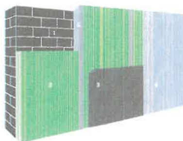
1. Buitengevel | 2. Isolatie | 3. Dampschermb | 4. Binnenaferking | 5. Stijl- en regelwerk (optioneel)
